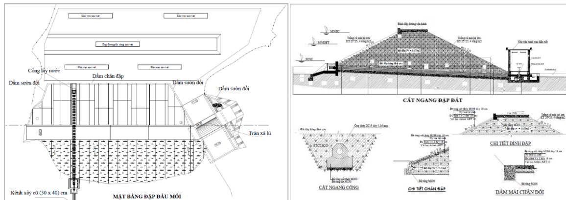
Hình 36. Bản vẽ thiết kế hồ chứa Bình Dân
