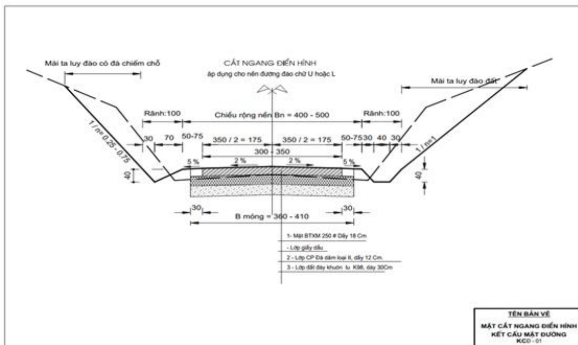
Hình 32. (Loại 1) Áp dụng cho rãnh thoát nước đất chữ U hoặc L
