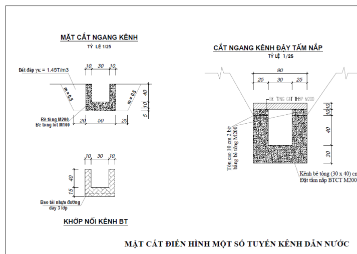
Hình 37. Mặt cắt ngang điển hình của kênh thủy lợi
