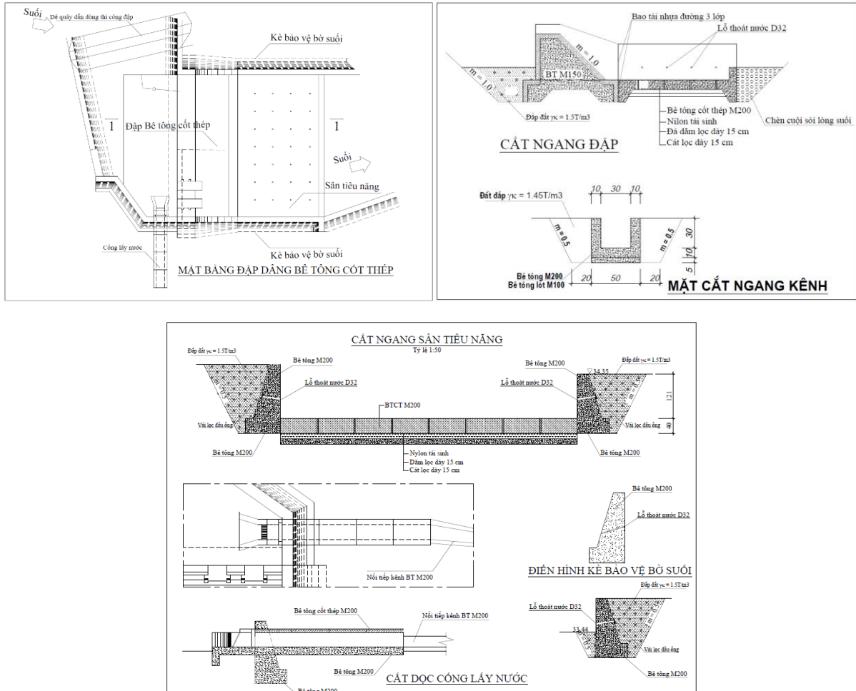
Hình 35. Bản vẽ thiết kế đập dâng Khẩu Lầu
