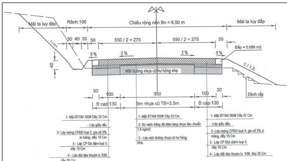
Hình 31. Mặt cắt điển hình đường liên xã
