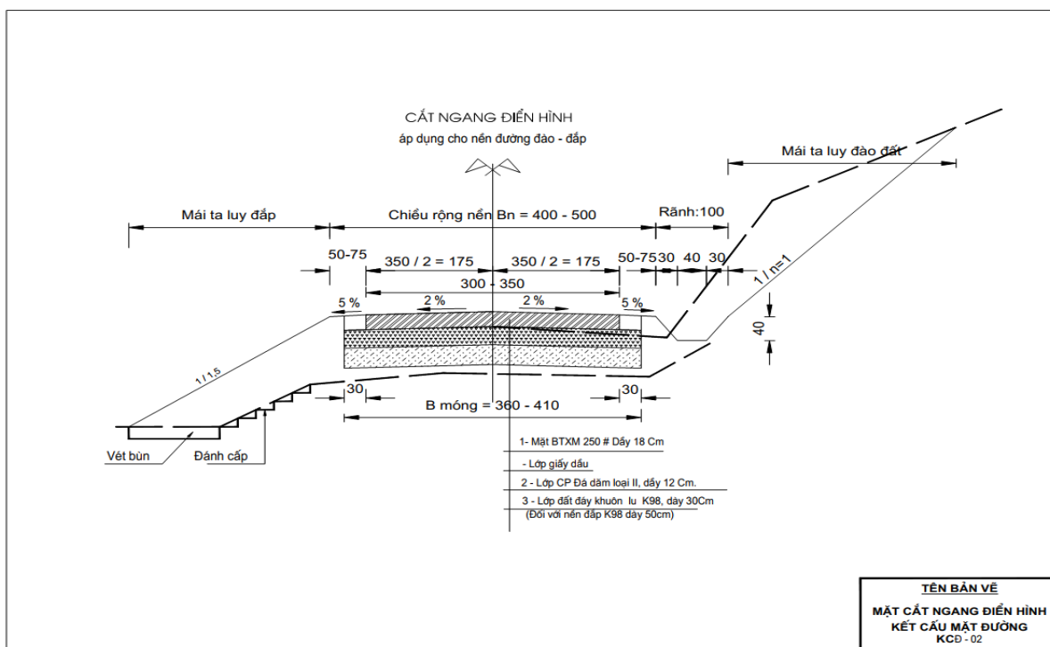
Hình 33. (Loại 2) Áp dụng cho nền đường đào - đắp
