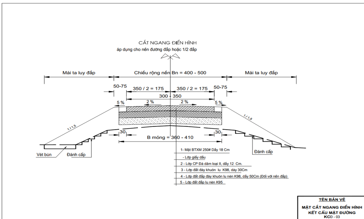
Hình 34. (Loại 3) Áp dụng cho nền đường đắp
